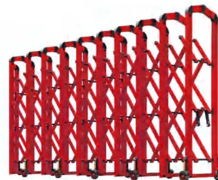
CX084 高速路障 high way road-block 最佳高度:1200mm 见光:400 包边:600
