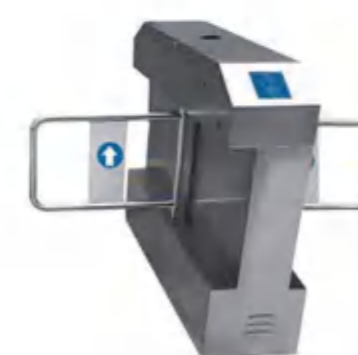
607A 双机芯摆闸
